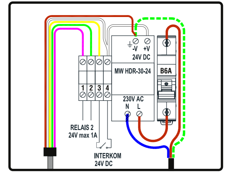
TESTEINHEIT UND NETZTEIL ANSCHLUSSPLAN
